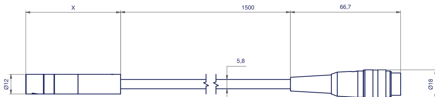
Zeichnung LED-Kopf HP
