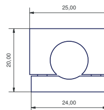
Halteblock LED-Kopf HP
